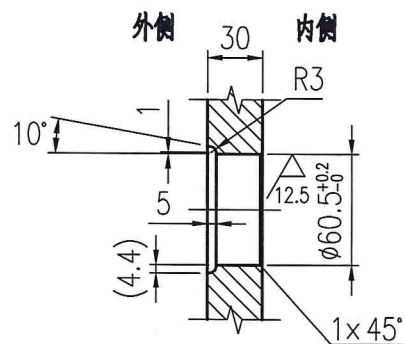
开孔详图
