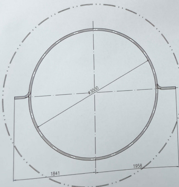
A向 不按比例
