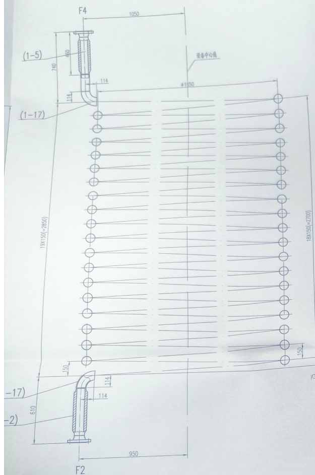
F2, F4盘管示意图 不按比例
