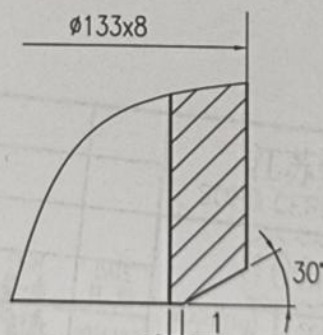
端面坡口详图
