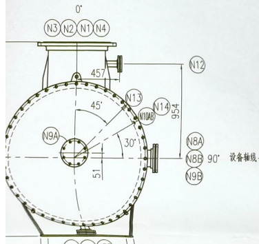
A向 A Direction 1:25
