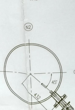
B-B 1:12
