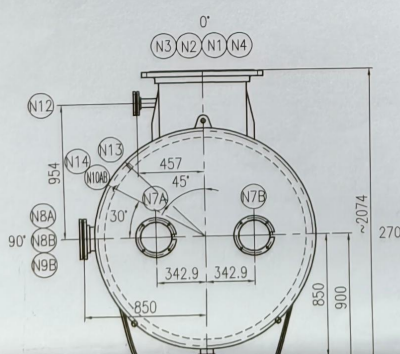
C向 C Direction 1:25
