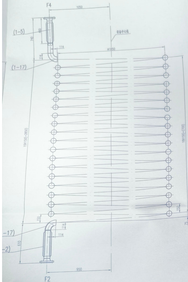
F2, F4盘管示意图 不按比例
