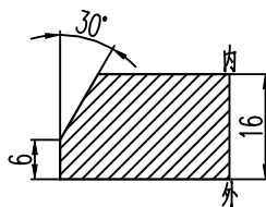
坡口1 (内坡口)
