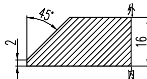
坡口2
